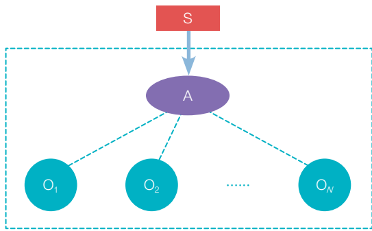
图3 多个观察者形成对微观系统的客观测量
